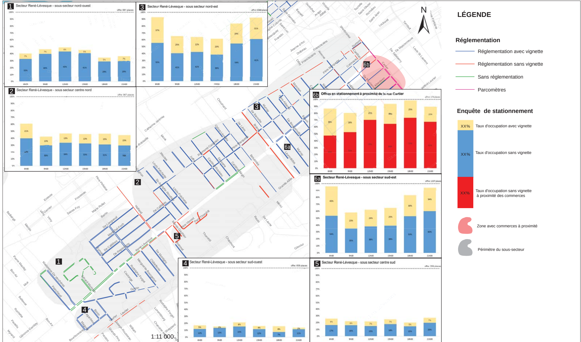
Figure A9-5 Relevé de stationnements Secteur René-Lévesque
